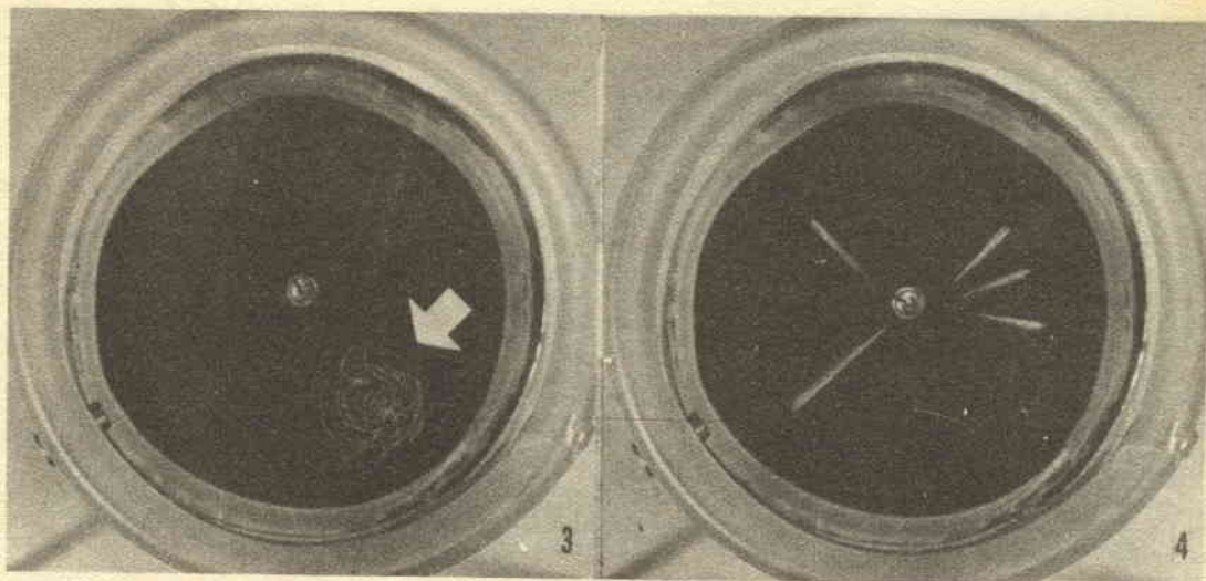
Foto 3 - La freccia indica la traccia di una particella rispettivamente prima, durante e dopo la colli- sione di questa con un'altra particella, eventualmente proveniente dal gas che riempie la camera a nebbia. La radiazione indicata è anche quella dei raggi cosmici, la nebbiolina appena percettibile è determinata da particelle beta che tendono a cadere verso il fondo della camera. Foto 4 - Le strisce di nebbia determinate da un frammento infinitesimale di un sale di mesotorio. La larghezza delle strisce è determinata dall'azione del campo elettrostatico per la eliminazione degli ioni che eccezionalmente viene lasciato inserito anche durante il funzionamento della camera proprio per la conduzione di que- sto esperimento.
