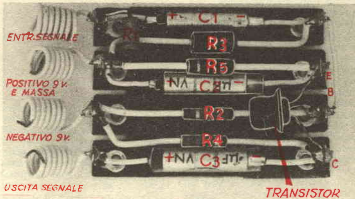
Foto illustrante la realizzazione pratica del complesso e la disposizione di tutti gli organi che lo compongono.
