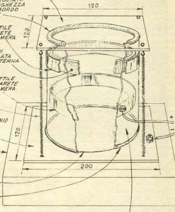
RECIPIENTE CILINDRICO DI PLEXIGLAS LUNGO 100, SPESSE 1,5 E DEL DIAMETRO DI 90
